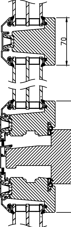
Vertikal- snitt karmpost
